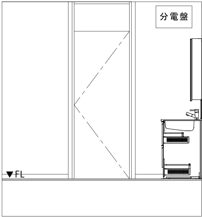
D 展開図
