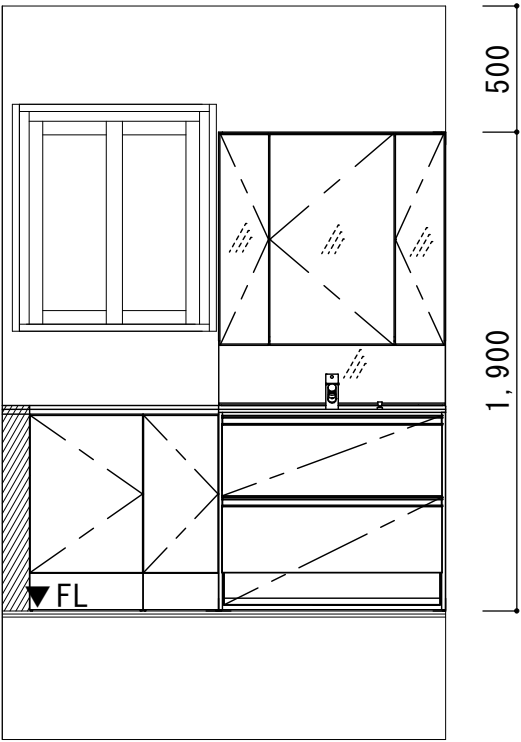
A 展開図
